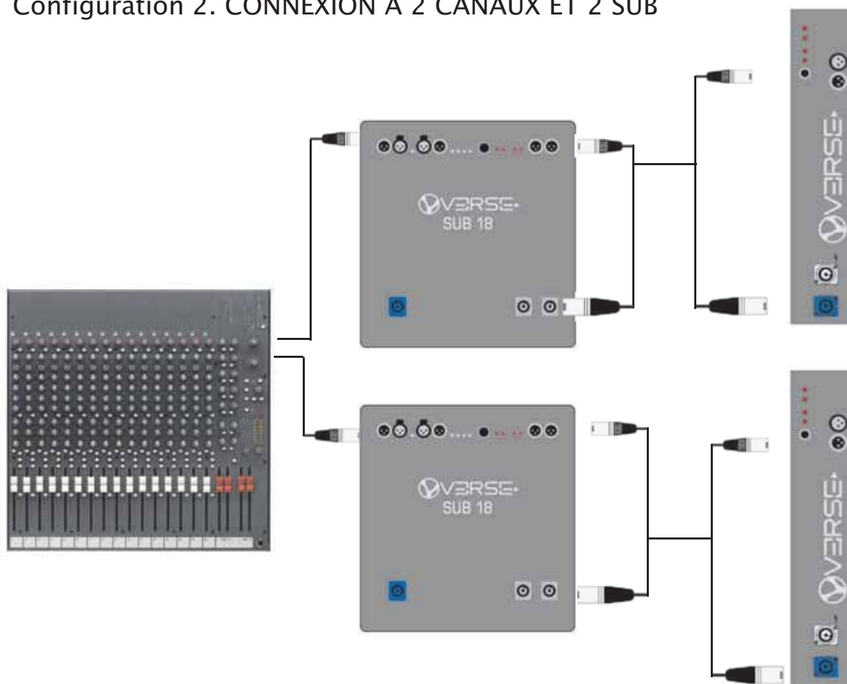
Configuration 2. CONNEXION À 2 CANAUX ET 2 SUB
